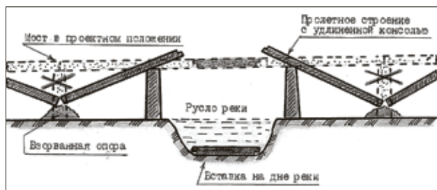
■ Благодаря схеме Авенира Овсянова даже неспециалисту понятно, как сборно-монокричный Пальмбургский мост стал «разводным»
